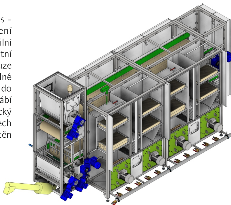
Modulární uspořádání sušárny
